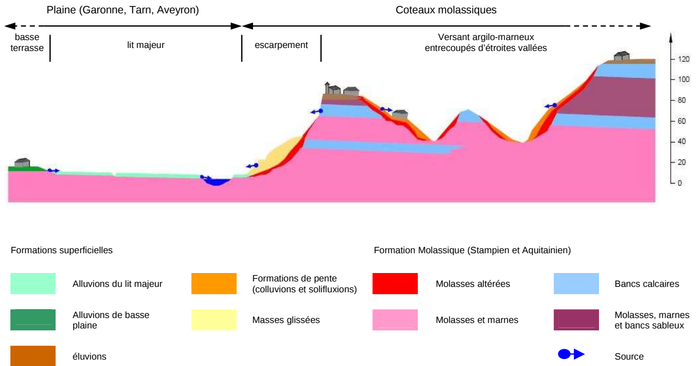
Figure 4 : Coupe géologique et géomorphologique schématisée
