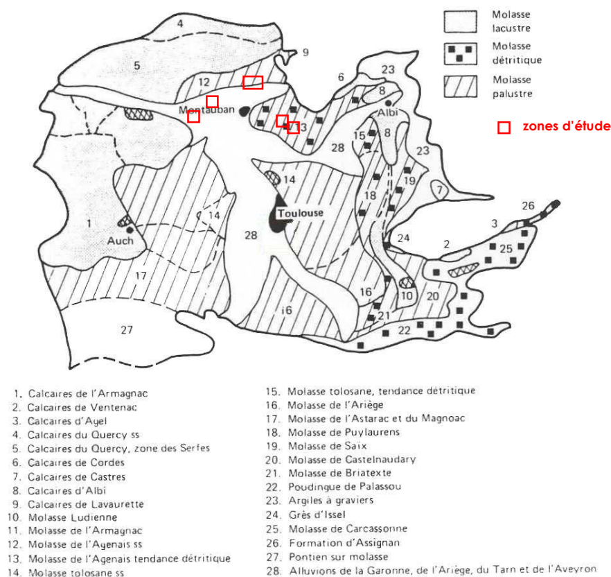
Figure 2 : Situation des Molasses* en Midi-Pyrénées
